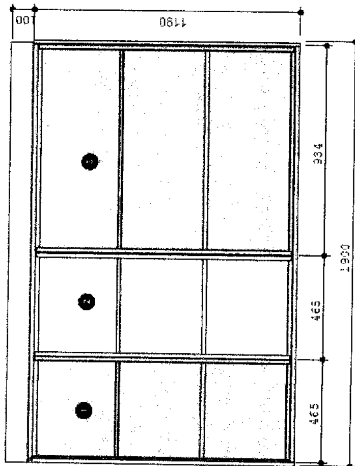
Vista Frontal Interna
