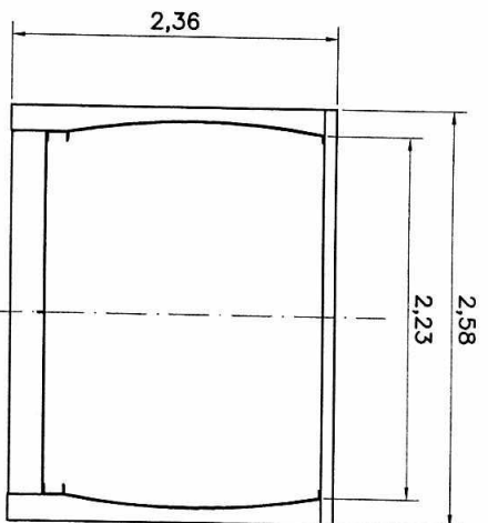
VISTA TRASEIRA CAIXA ARMAZENAGEM ESCALA 1:30
